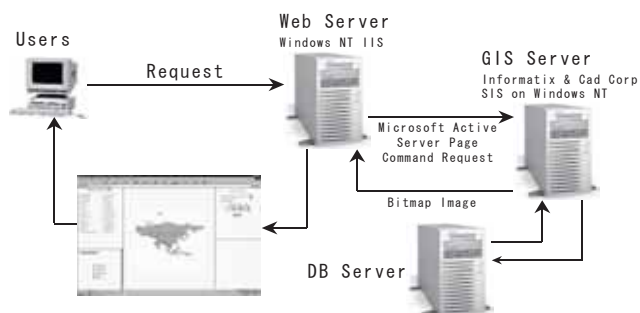
図2-7-2-4-1 VENTENにおける処理のフロー
