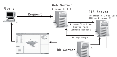
図2-7-2-4-1 VENTENにおける処理のフロー
